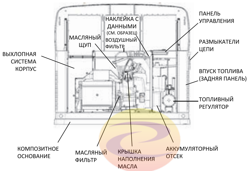
Рисунок 2-1: Двигатель GN-530, блок 8 кВА
